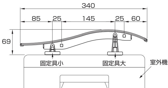
寸法図(mm)
