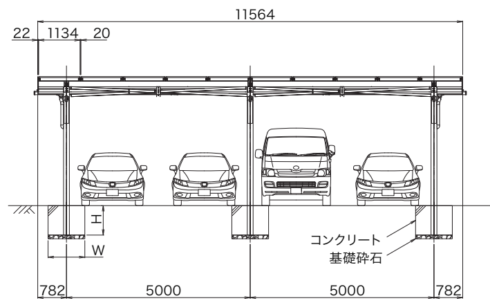
正面図
