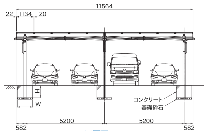
正面図
