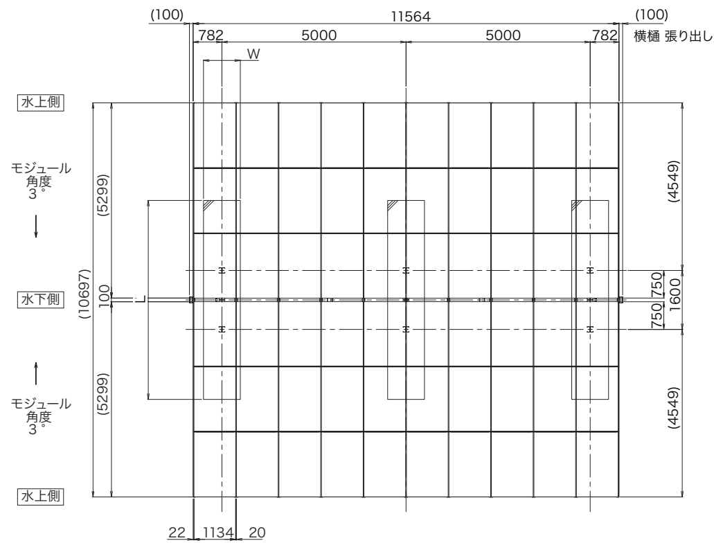
平面図
