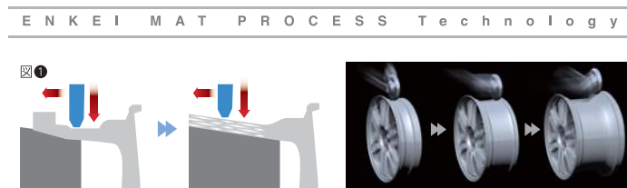
MAT 処理前の組織 MAT 処理後の組織 マンドレル(芯金)型に固定し、回転させながらローラーによって圧延加工を施すとアルミ合金の金属組織に、鍛造製法の特徴である「鍛流線」が現れます。
