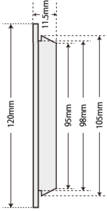
調湿プロテクター (シリコン部) 寸法図
