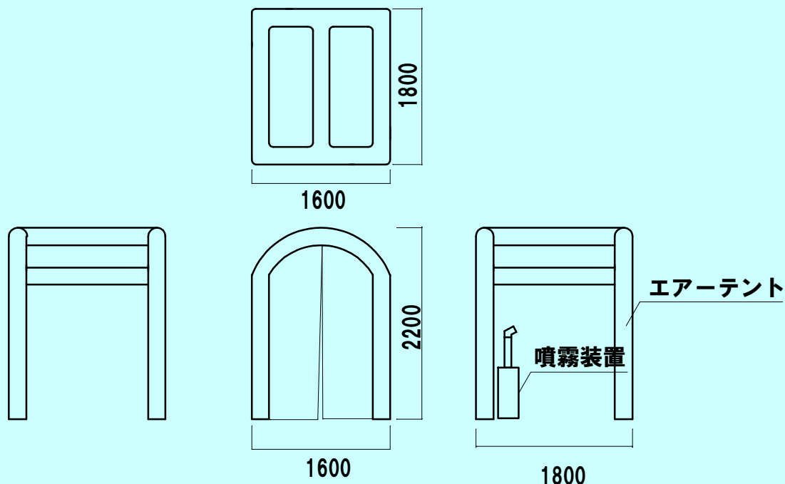
【ポータブルタイプ外形寸法図】
