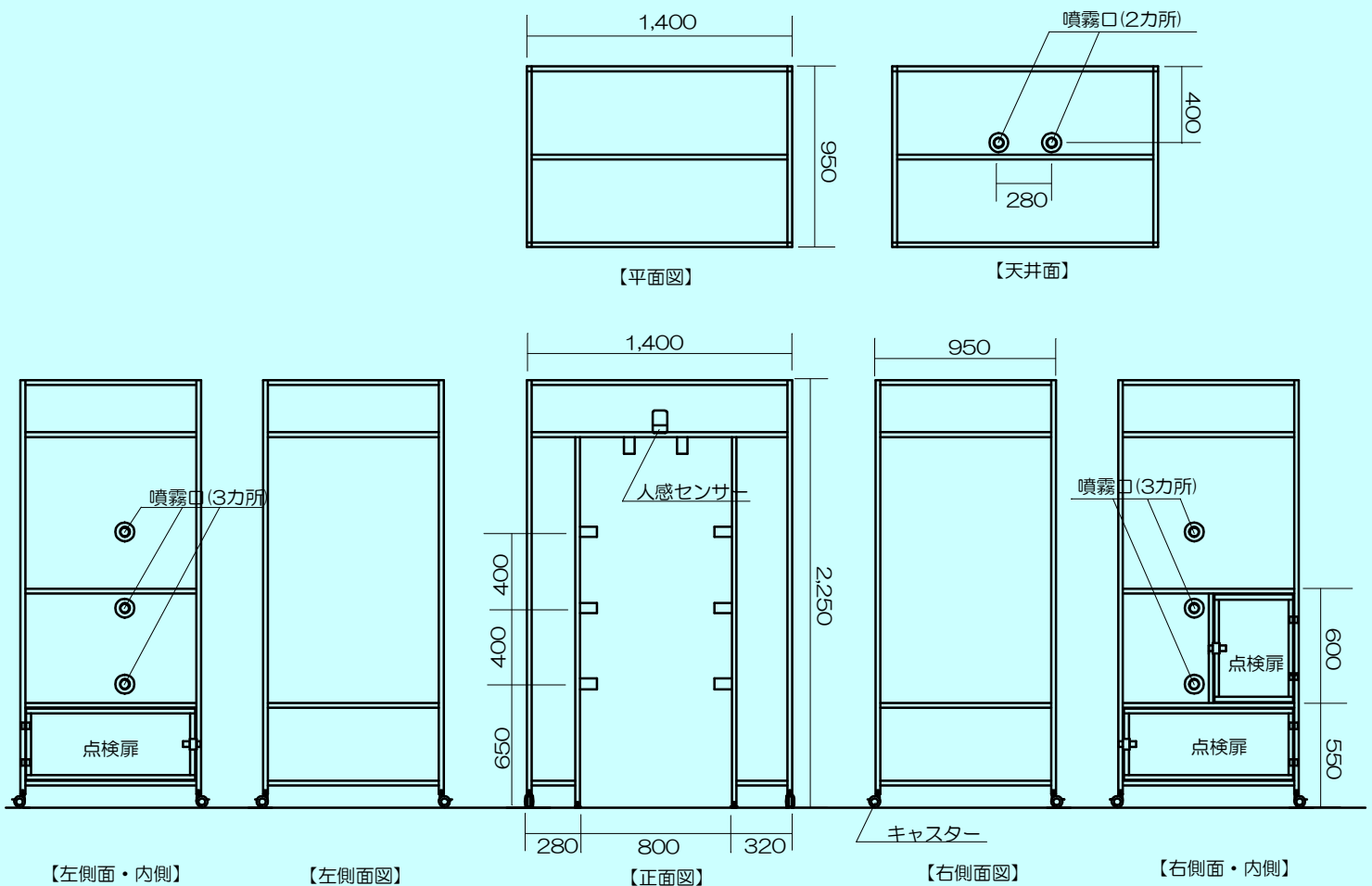
【スタンダードタイプ外形寸法・機能説明図】
