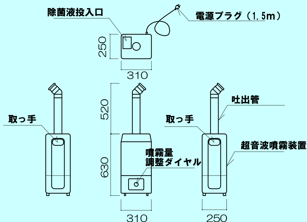
【超音波噴霧装置外形寸法図】
