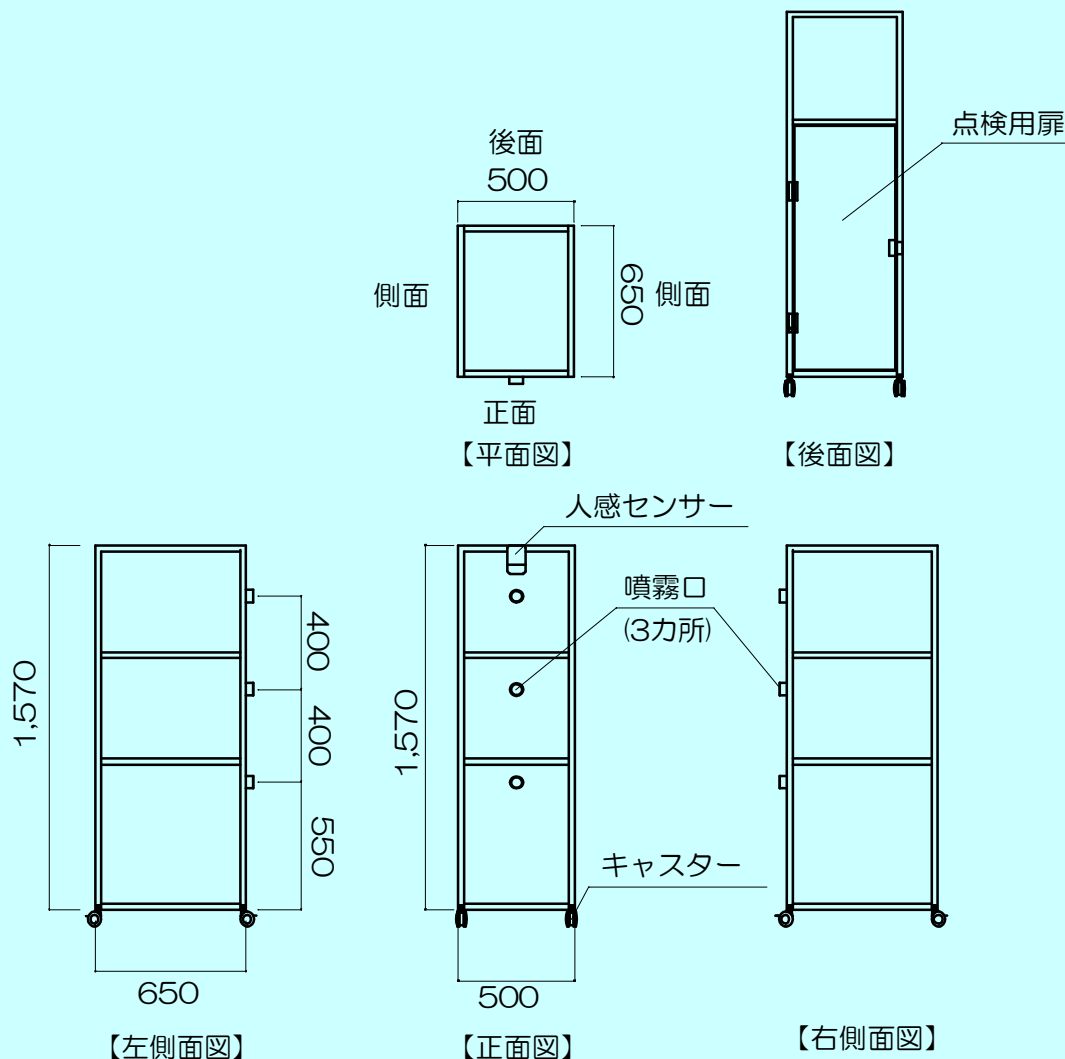
【タワータイプ外形寸法・機能説明図】
