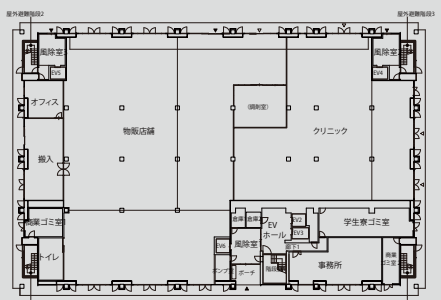
1階平面図
