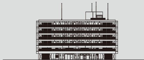
南立面図
