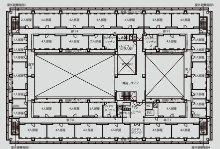
6階平面図
