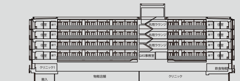
a断面
