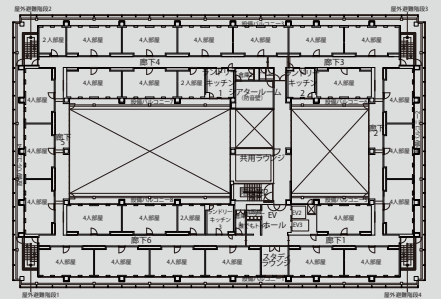
4階平面図
