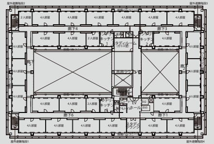
5階平面図
